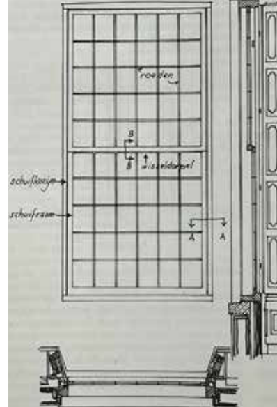
Schets van de aanpak van een schuifvenster (bron: Haslinghuis – Bouwkundige termen – 1997)
