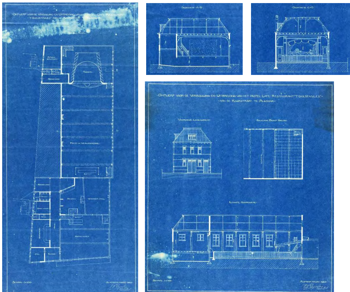
Afb.1.9a Blauwdrukken van P.N. Leguit voor verbouwing en nieuwbouw van de schouwburg, 1923
