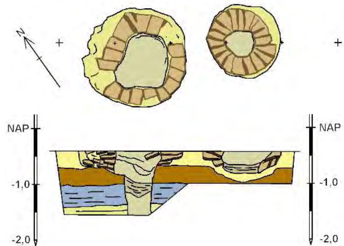
Afb.2.10 Plattegrond en doorsneden van waterputten 1C (links) en 1D (rechts), 1:150
