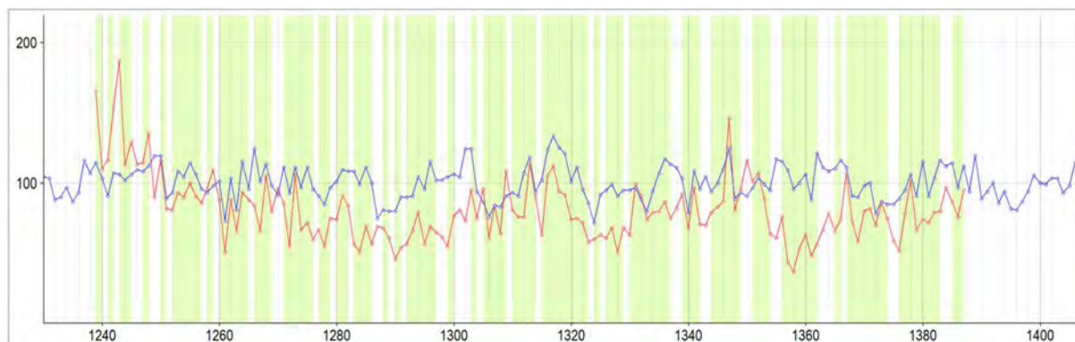
Afb.5 Visuele overeenkomst tussen referentiekalender PLOPOM01 (blauw) en 23AK0071 (rood). X-as: kalenderjaren; Y-as: jaarringbreedte in mm *10 -2 ; Lichtgroen: intervallen van parallelle ringbreedtevariaties.
