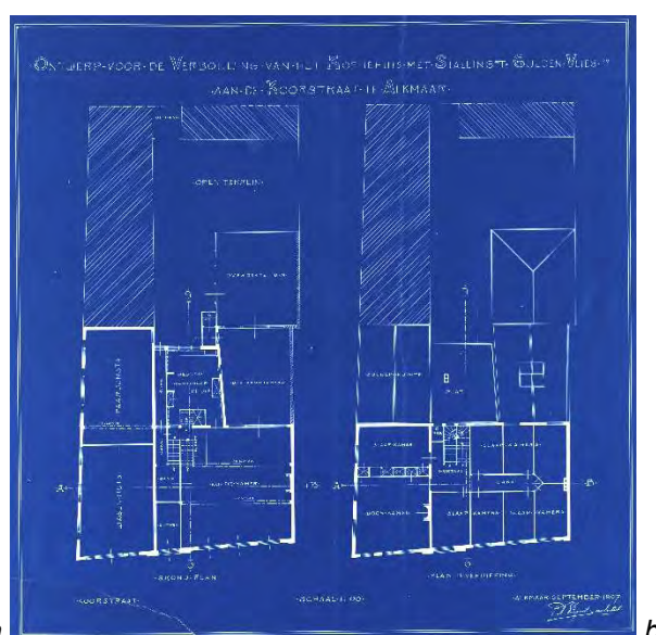
Afb.1.8 a-b. Bouwtekeningen van P.N. Leguit voor de nieuwbouw, 1907; c. bestaand pand bij de aanvraag in 1923 (Regionaal Archief Alkmaar)
