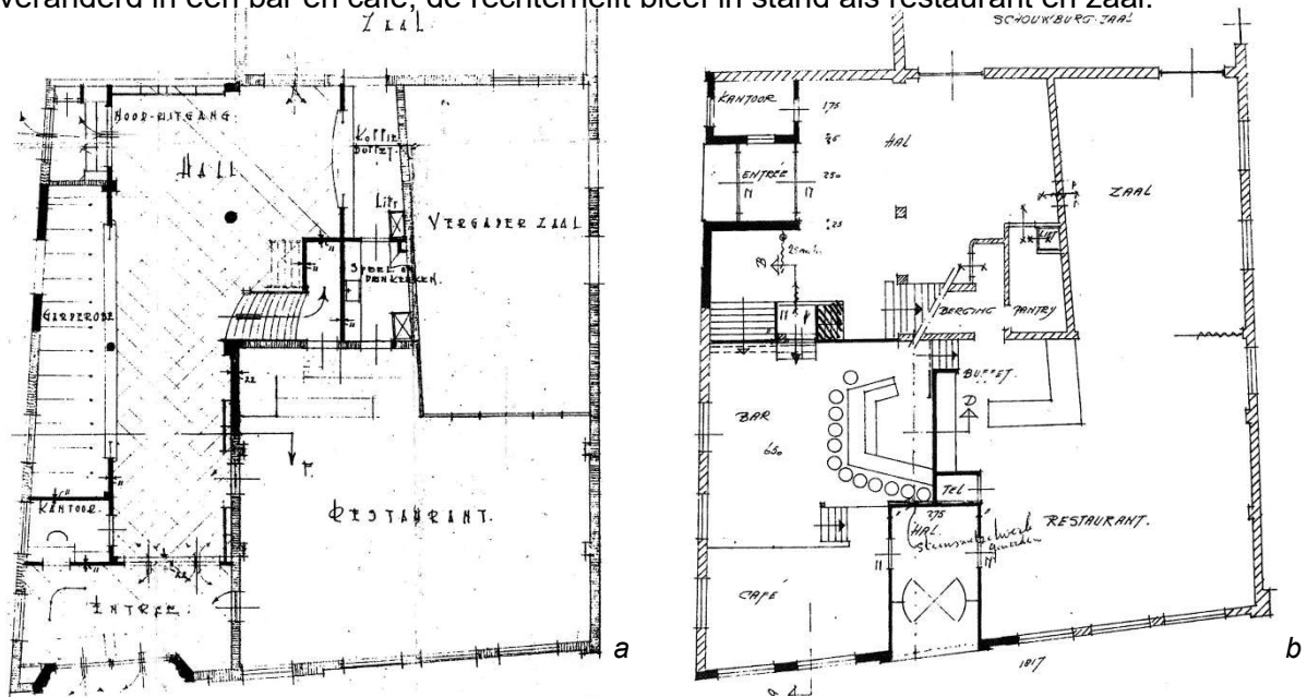
Afb. 1.10ab Bouwtekeningen van verbouwingen in 1951 en 1971 (Stierp-Impink e.a. 1999)
