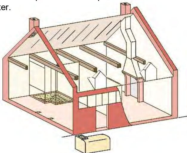
Afb.2.26a Reconstructie van de twee-kamers-onder-één-dak op Kad.A828
