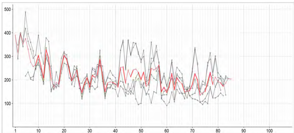
Afb.2 Visuele overeenkomst tussen jaarringenpatroon van duig 1, 2, 3, 4 en 8 (tonput S1059, vnr. 41) (grijs) tot gemiddelde boomgroep 23AK_1_2_3_4_8_TG (rood). X-as: aantal jaarirngen; Y-as: jaarringbreedte in mm *10-2.
