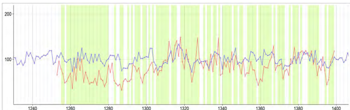
Afb.4 Visuele overeenkomst tussen referentiekalender PLOPOM01 (blauw) en 23AK0061 (rood). X-as: kalenderjaren; Y-as: jaarringbreedte in mm *10-2; Lichtgroen: intervallen van parallelle ringbreedtevariatiies.
